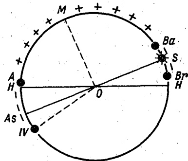
Рис. 3.2. Нейтральные точки небосвода.
