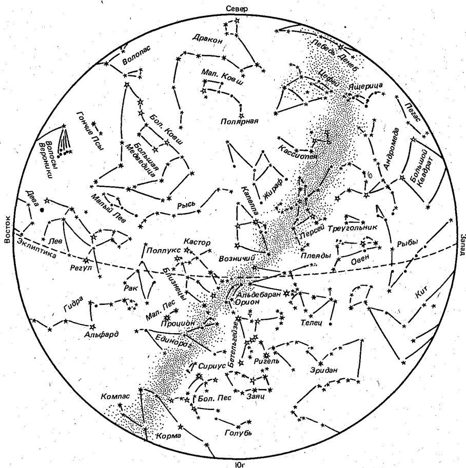
Рис. 15.1. Созвездия зимнего неба на широте 40° С Из книги Г. Рея „Звезды“.
