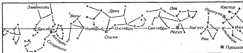
Рис. 15.2. Годовое движение Солнца по 12 созвездиям Зодиак:
