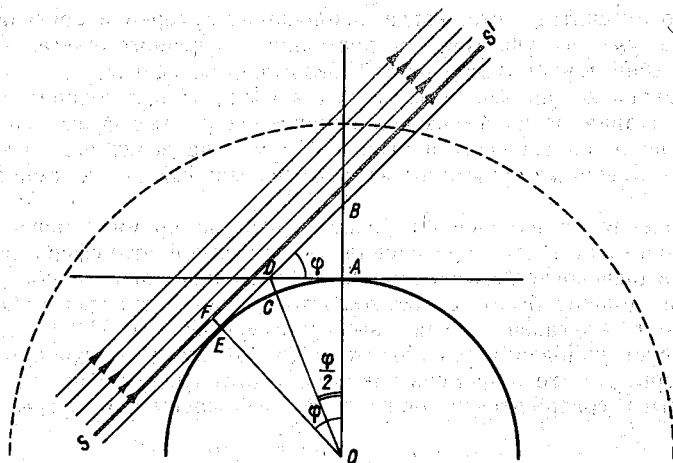
Рис. 13.1. Освещение земной поверхности в сумерки.
