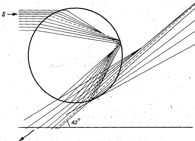
Рис. 5.2. Преломление пучка световых лучей в капле.
