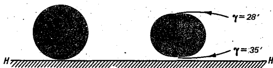
Рис. 10.2. Сплющивание диска Солнца и Луны у горизонта.
