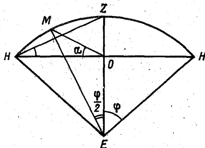
Рис. 3.3. Сплюснутость небесного свода.
