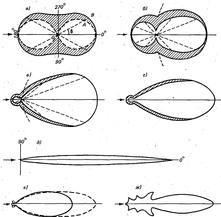
Рис. 2.2. Индикатрисы рассеяния.
