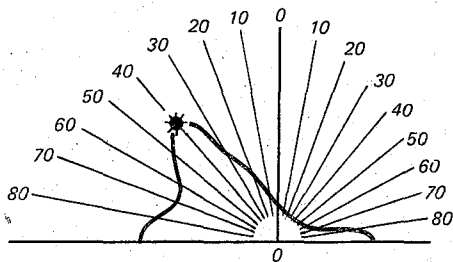
Рис. 3.1. Распределение яркости по небосводу в вертикале Солнца.
