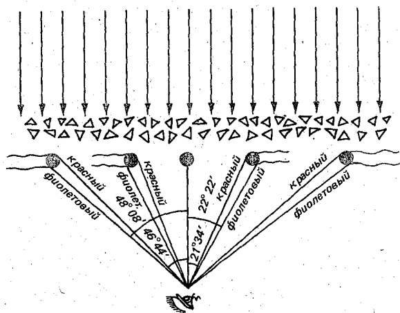
Рис. 6.4. К образованию ложных солнц и гало радиусом 22^\circ и 46^\circ .
