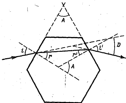
Рис. 6.3. Ход светового луча в ледяном кристалле.
