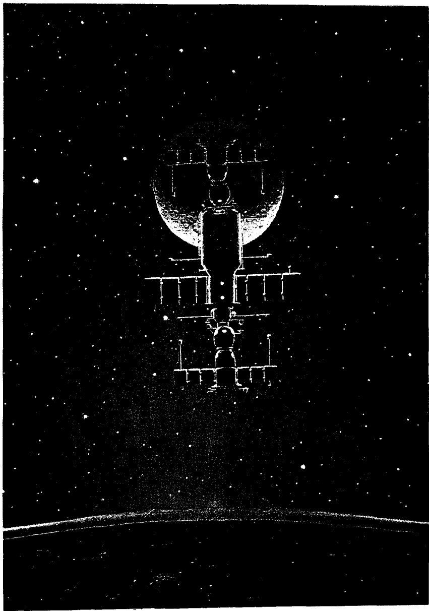
Зодиакальный свет, наблюдаемый из космоса. (Фото А. Кулешова по рис. художника А. К. Соколова)
