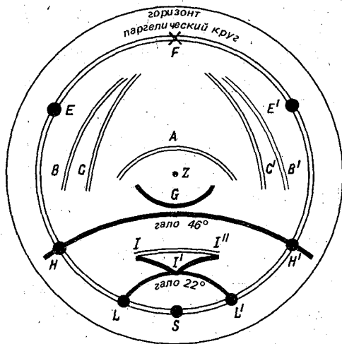
Рис. 6.10. Схема сложного комплекса гало, наблюдавшегося на станции Амундсен-Скотт 28 января 1977 г. А. Хоганом.
