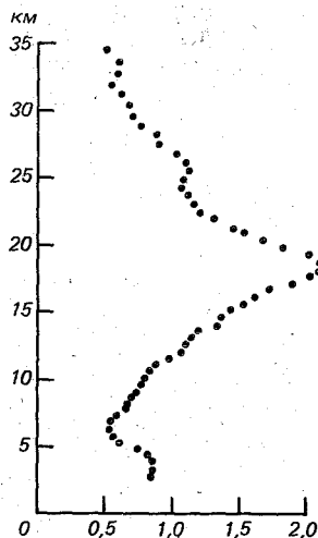
Рис. 7.1. Изменение с высотой средних коэффициентов аэрозольного рассеяния после извержения вулкана Агунг.
