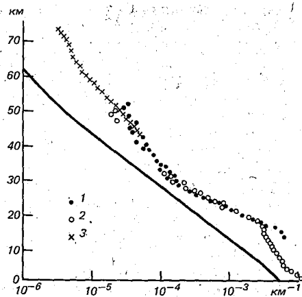
Рис. 7.2. Вертикальные профили объемных коэффициентов рассеяния атмосферы, полученные различными методами: 1 — наблюдение с пилотируемого космического корабля „Союз-3“, 2 — прожекторное зондирование, 3 — сумеречный метод. Сплошная кривая — значения коэффициента молекулярного рассеяния.
