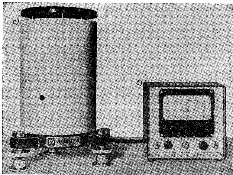
Рис. 1. Общий вид инспекторского манометра абсолютного давления ИМАД-4М (а) и индикатор пульты (б).
