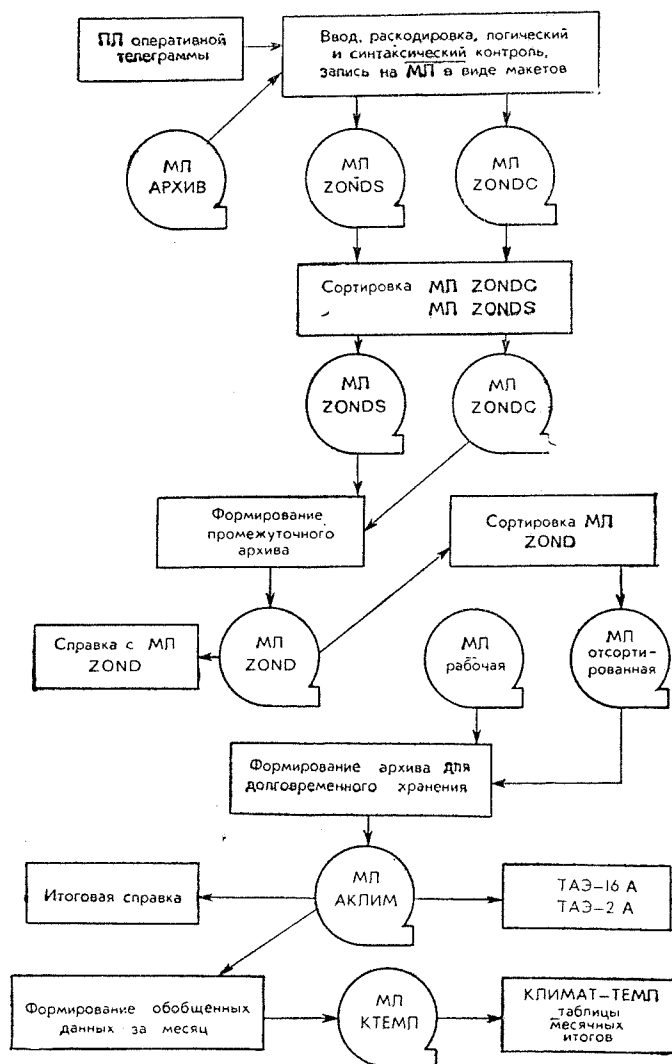
Рис. 1. Схема обработки аэрологической информации на ЭВМ «Минск-32»
