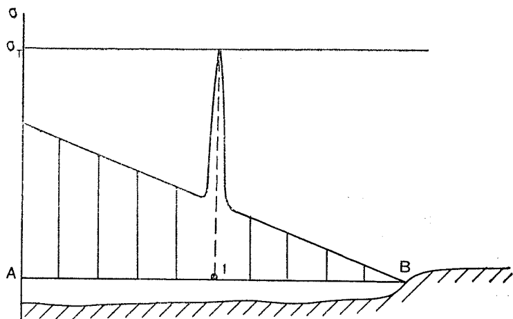
Рис. 1. Эпюра напряжений в припае при постановке судна в точке 1: \sigma_T — напряжение текучести морского льда; АВ — припай
