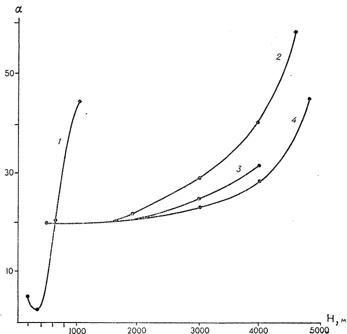
Рис. 1. Эпюры углов \alpha отклонения троса от вертикали в зависимости от глубины H по данным инструментальных наблюдений на ПБС:
