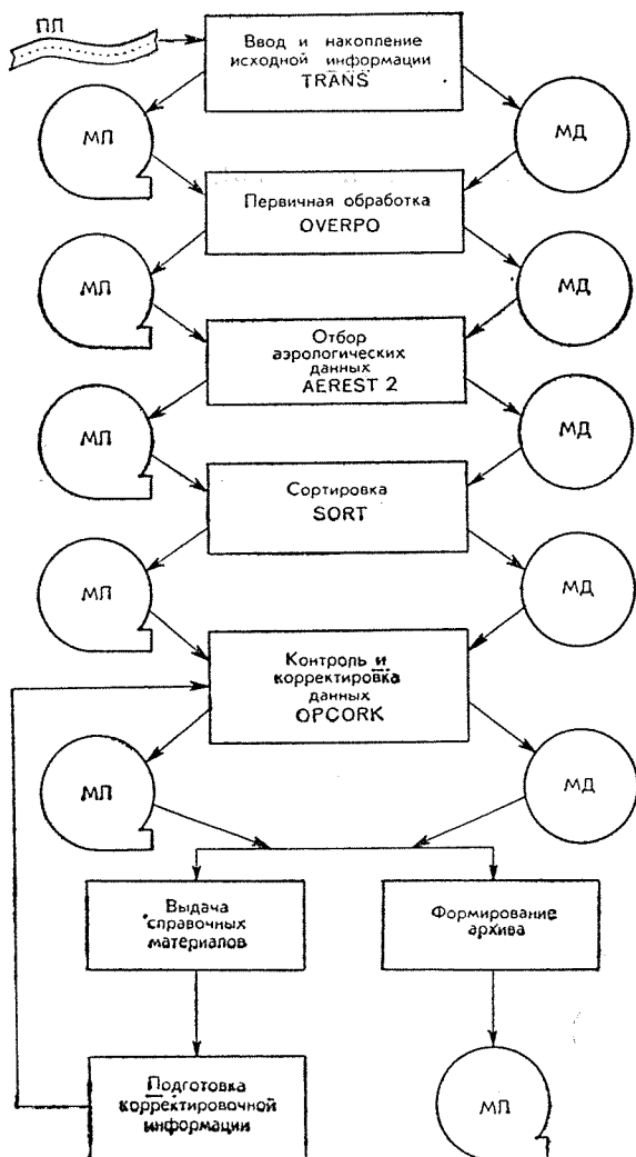
Рис. 2. Обработка судовой аэрологической информации на ЭВМ серии ЕС
