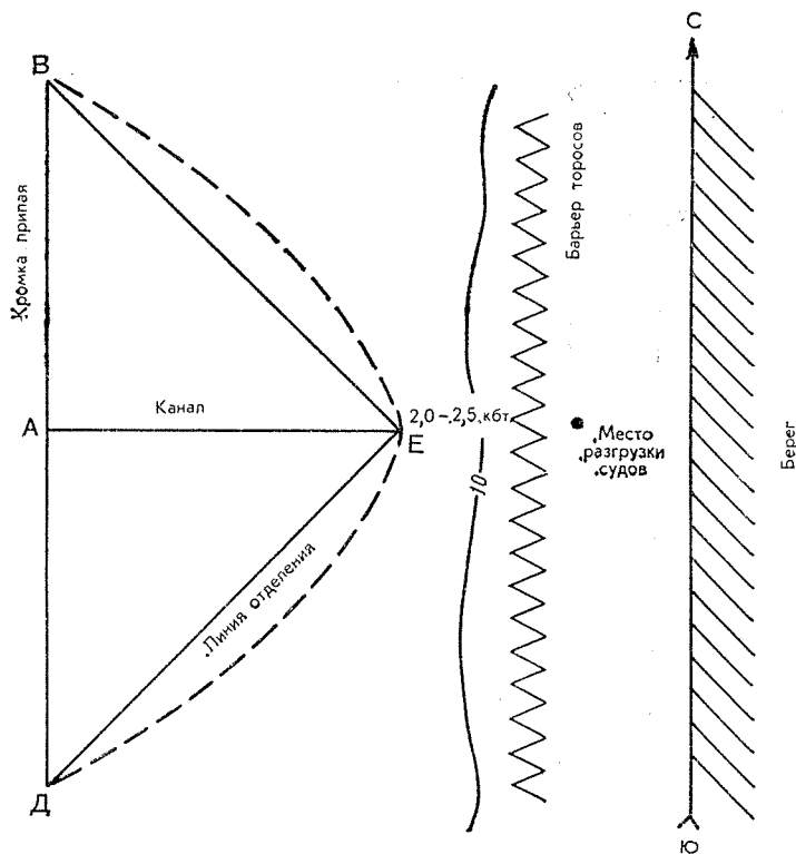
Рис. 3. Схема отделения припая ледоколом
