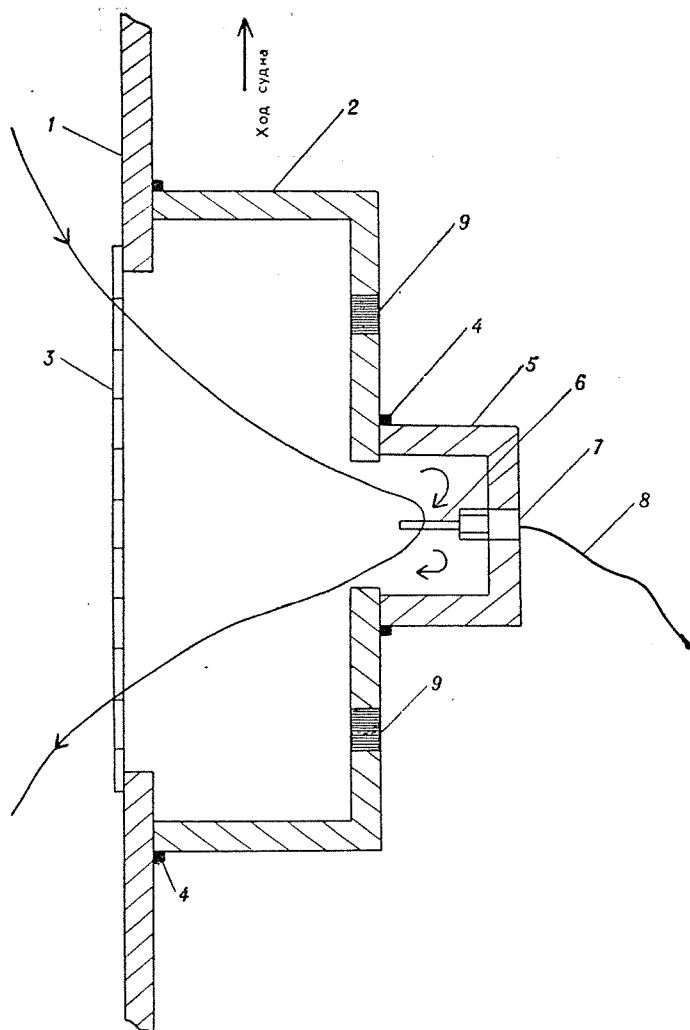
Рис. 1. Схема установки термометра сопротивления в кингстонной коробке:
