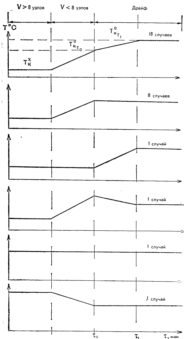
Рис. 2. Характер изменения ТПСВ при различных режимах плавания судна Тип (18 случаев) — средний и наиболее часто встречающийся
