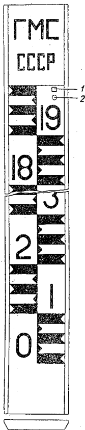
Рис. 10. Рейка водомерная постоянная деревянная.
