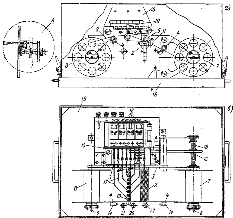
Рис. 29. Хронограф.
