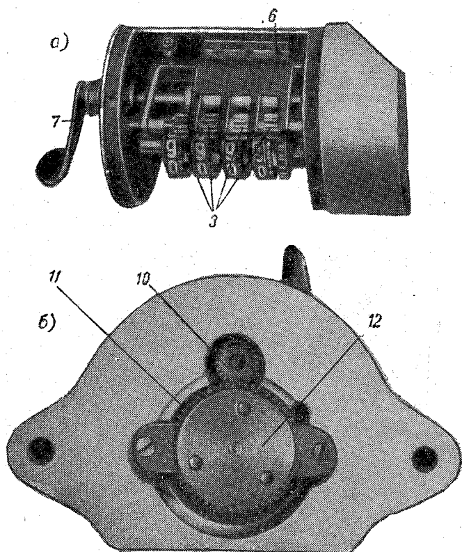
Рис. 54. Счетчик со сбросом на ноль (С-52-М) (вид сверху а и со стороны соединительной муфты б ).
