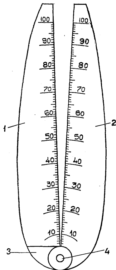
Рис. 65. Пропорциональный делитель.
