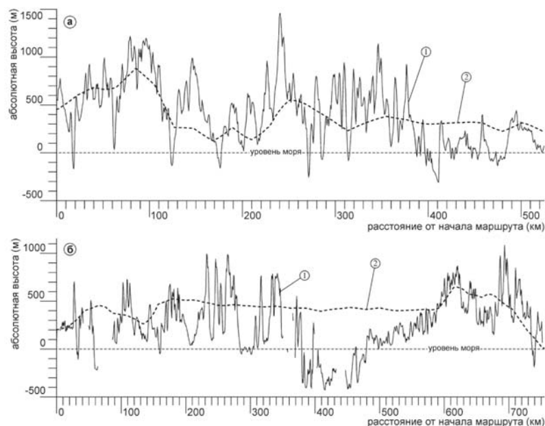
Рис. 4. Сравнение высот подледной поверхности по профилям (54)VK (а) и (54)КСТ (б) и карты BEDMAP:
