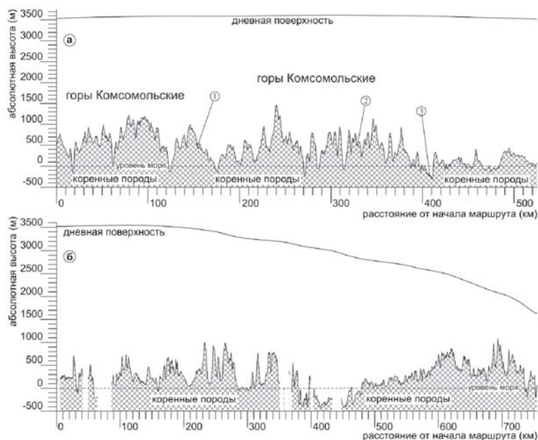
Рис. 3. Разрезы ледникового покрова по маршрутам (54)УК (а) и (54)КСТ (б). Цифрами показаны обсуждаемые в тексте подледниковые водоемы
